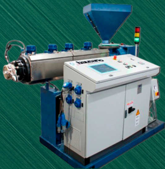
EXTRUSORAS DE UN HUSILLO
